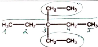
3,3-diethylpentane
